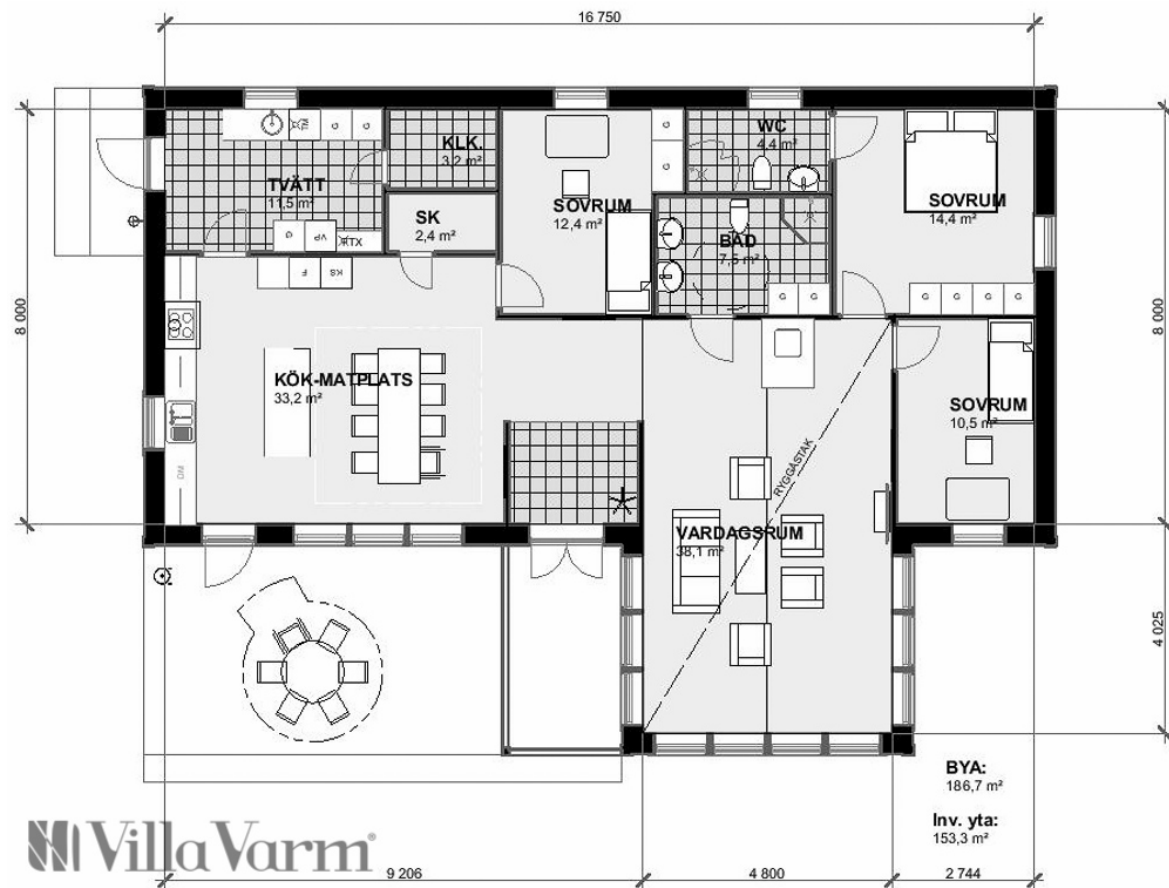
Planlösning Villa Hällfors
