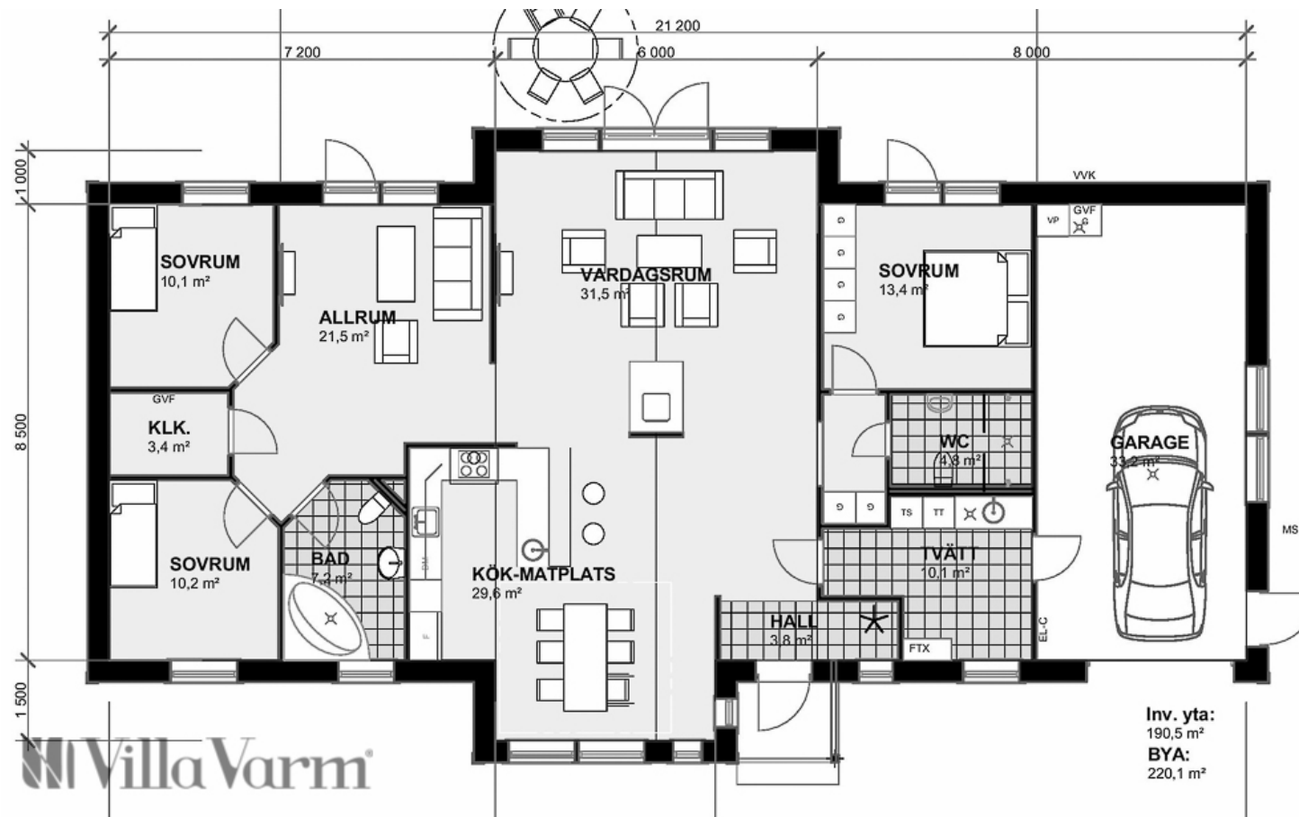
Planlösning Villa Furuvik
