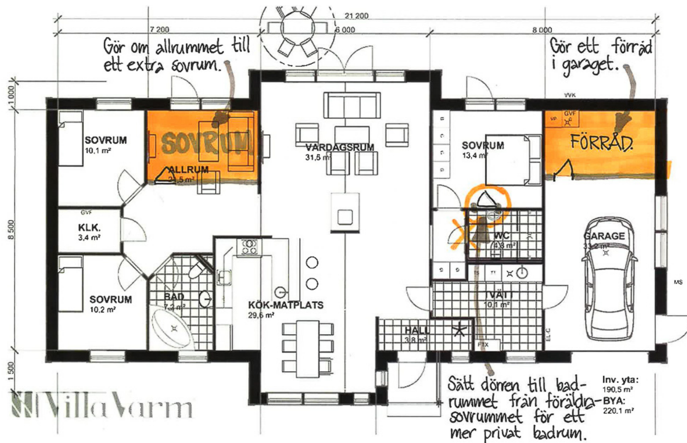
Ändring planlösning Villa Furuvik
