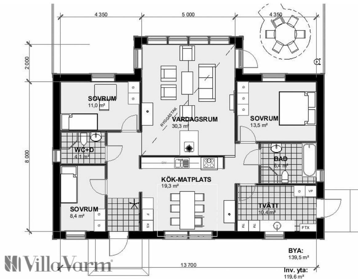
Planlösning Villa Backa
